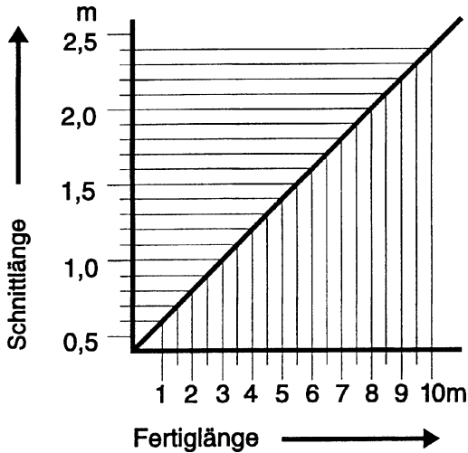
Diagramm zur Ermittlung der Schnittlänge von Knick- und Scheuerschutzfedern
