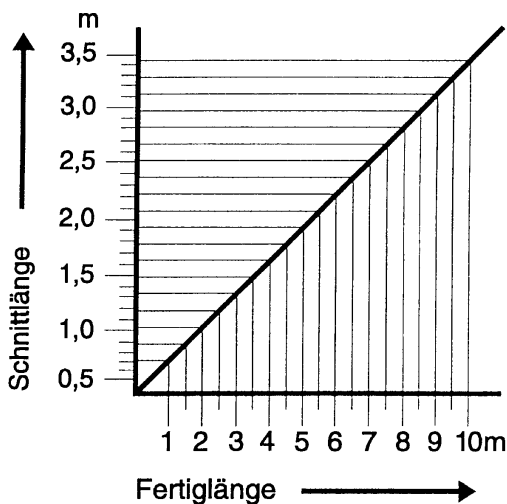
Diagramm zur Ermittlung der Schnittlänge von Knick- und Scheuerschutzfedern
