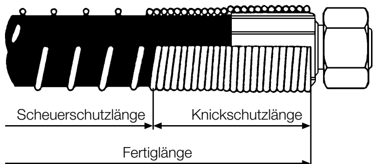
Diagramm zur Ermittlung der Schnittlänge von Knick- und Scheuerschutzfedern
